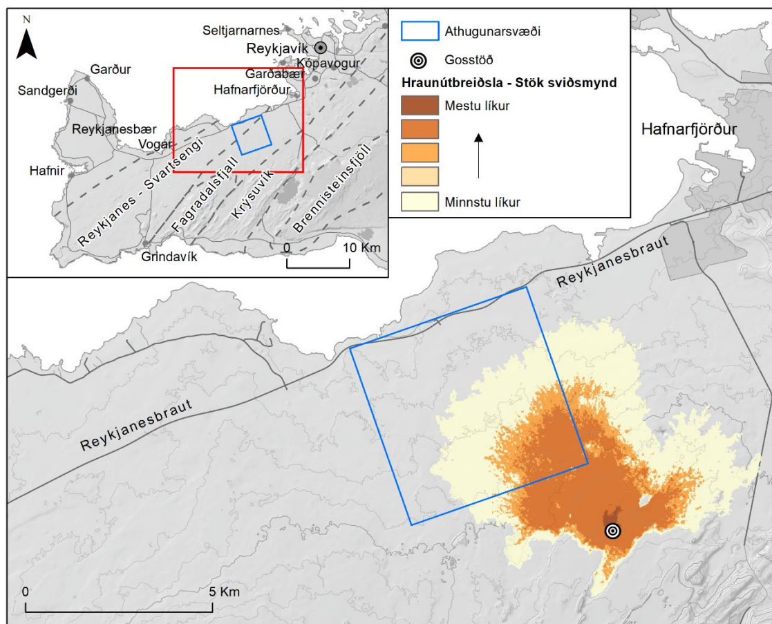
Mynd 6: Stök sviðsmynd (sbr. mynd 7 í viðauki nr. 8) hermds meðalstórs goss (0,3 km 3 ) með stutta rennislengd (5 km, sjá texta). Mesta hraunflæði í yfirstandandi jarðeldum á Reykjaneskaga er um 0,15 km 3 skv. minnisblaði Veðurstofu Íslands (viðauki nr. 11).
